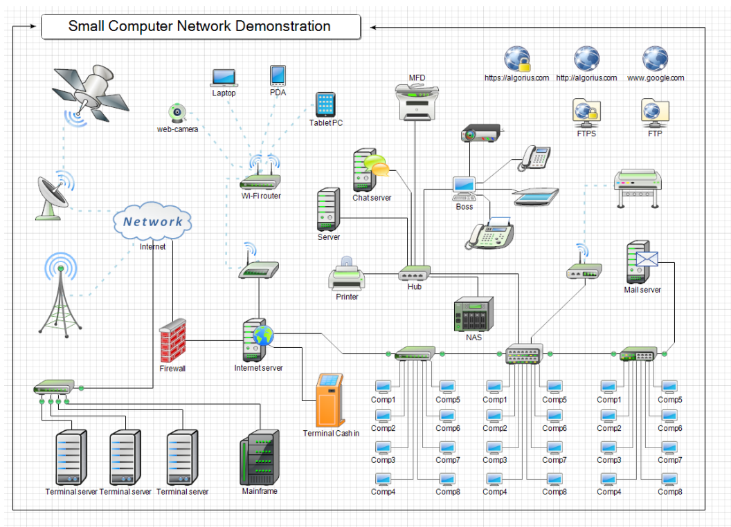
Рисунок 1 – Пример графического представления логической топологии сети
